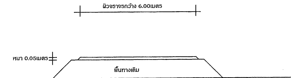
รูปตัดโครงการปรับปรุงถนนลาดยาง
