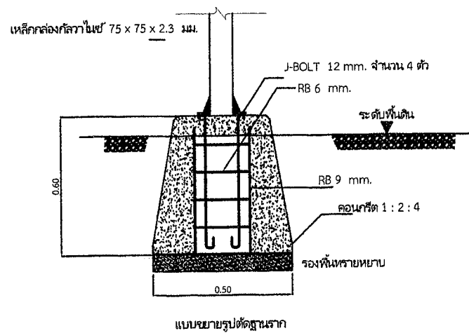
แบบขยายรูปตัดฐานราก
