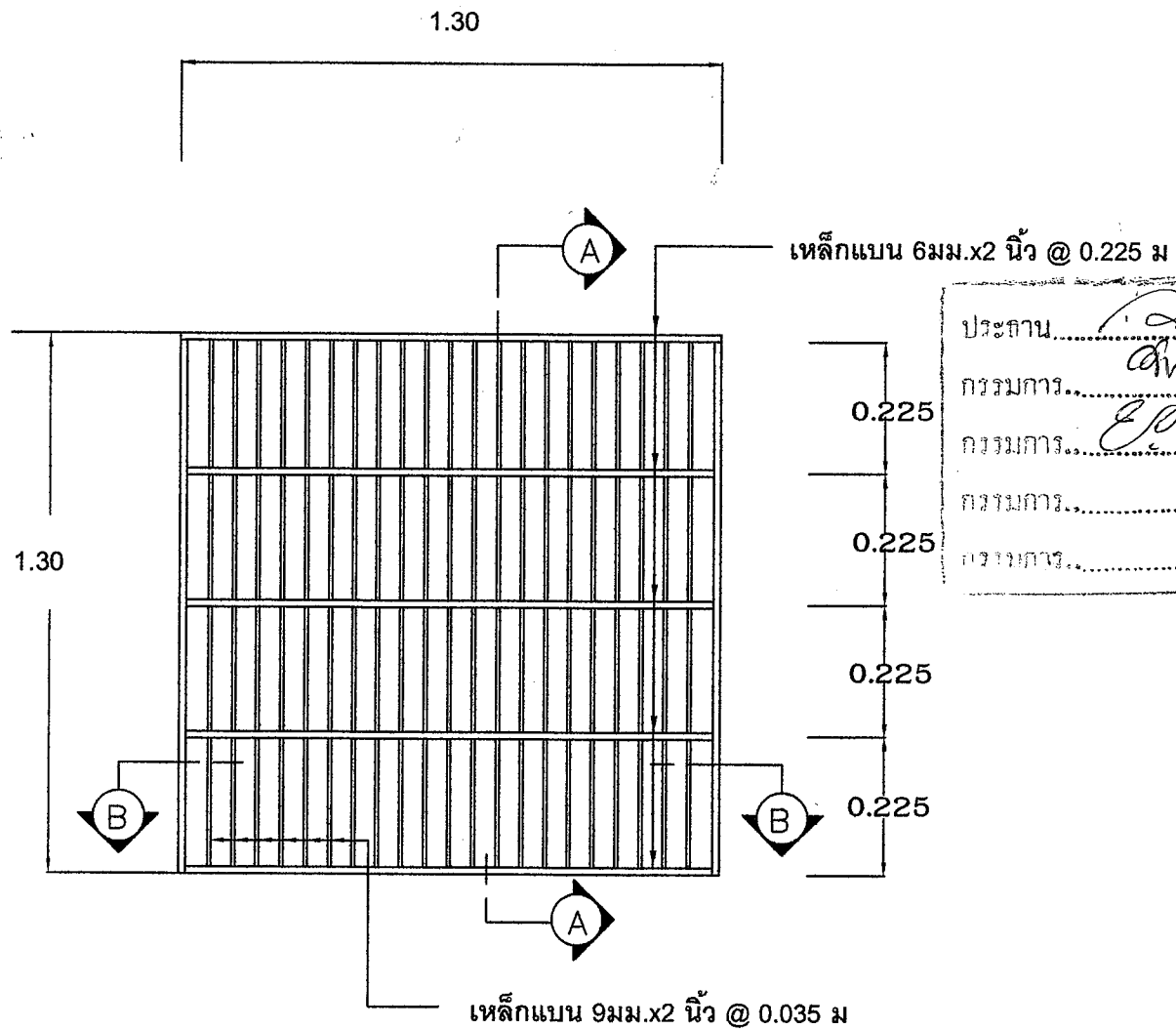
รูปแสดงเหล็กบ่อกักน้ำ
